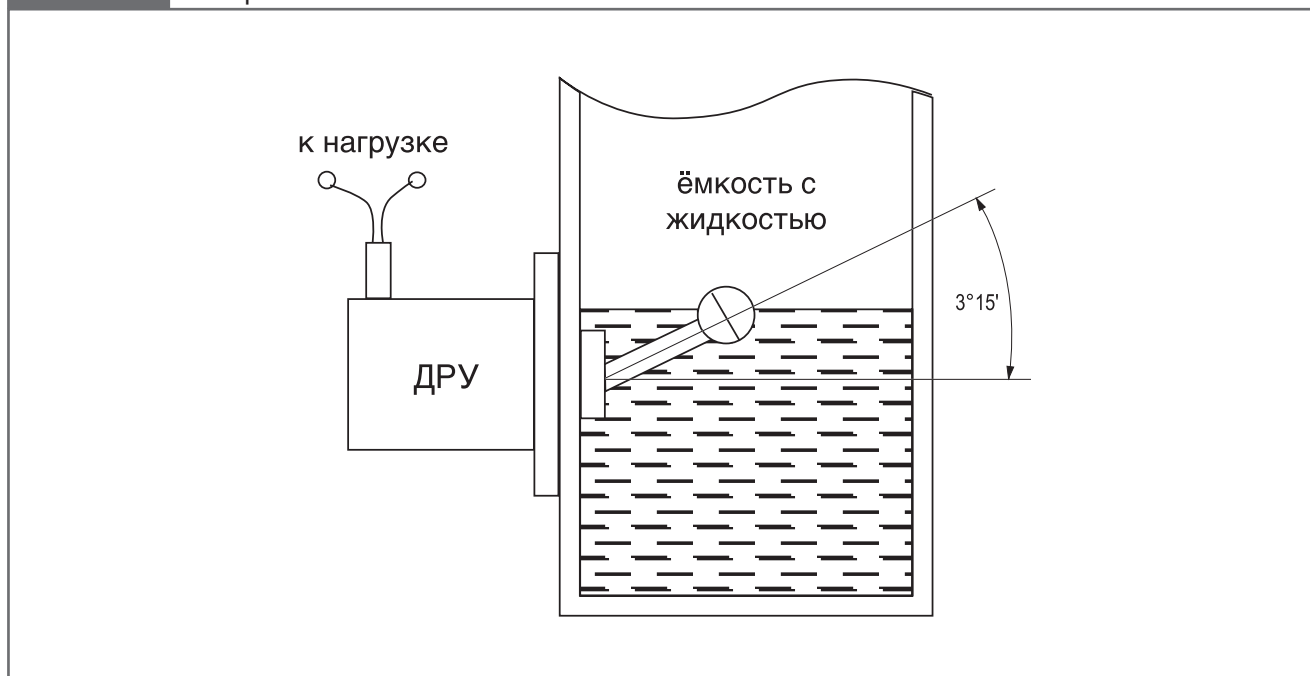
Вариант монтажа.
